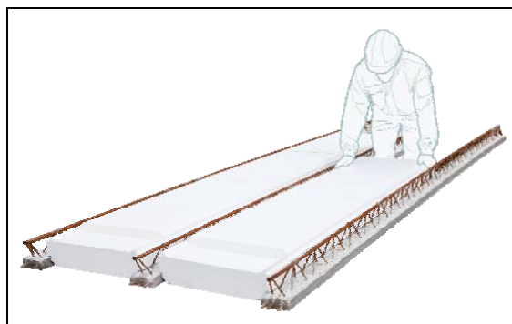
Poutrelles RAID SH et entrevous OPTIRAID®
