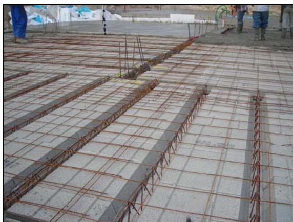
Poutrelles RAID SH et entrevous béton
